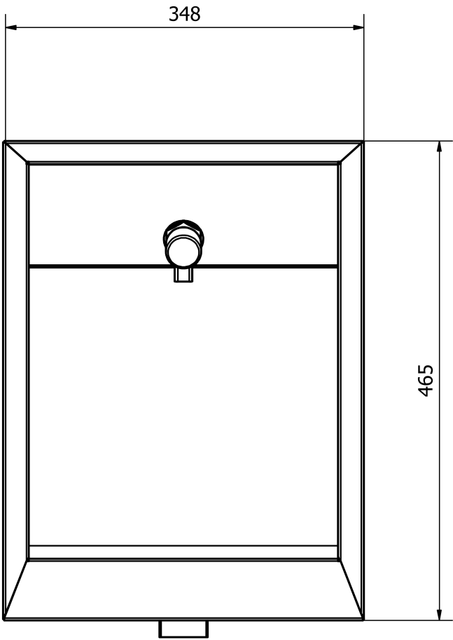
FRONT ( 1 : 4 )
