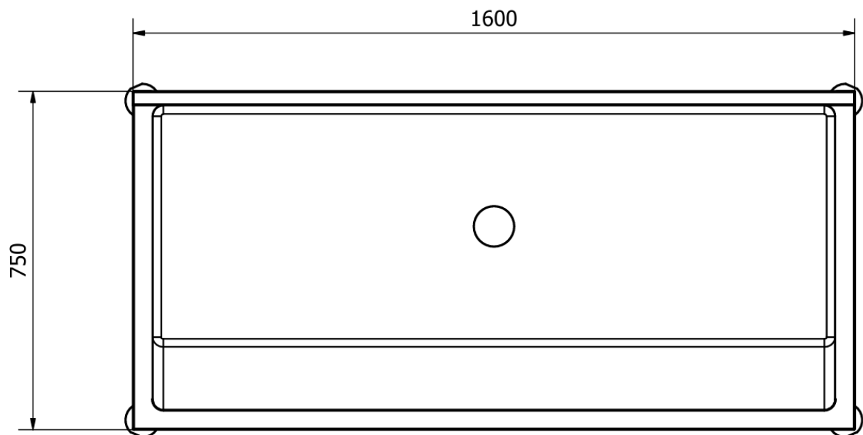
TOP
