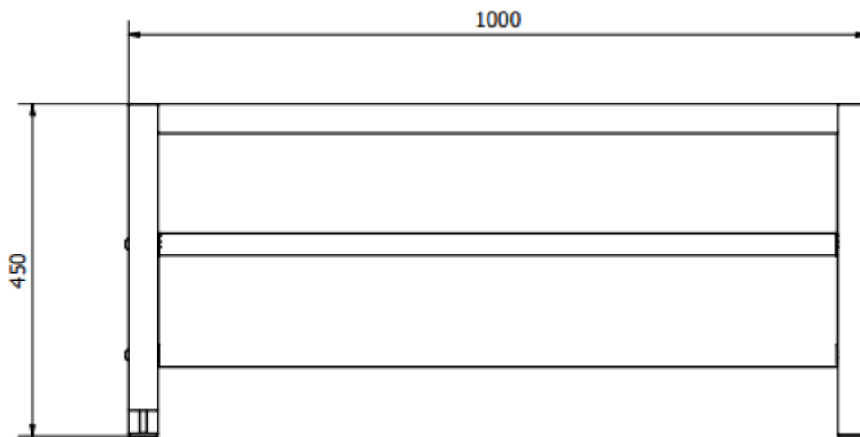
FRONT ( 1 : 6 )
